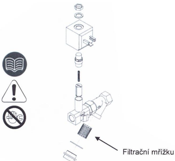
Čištění sítka ventilu odvaděče kondenzátu
